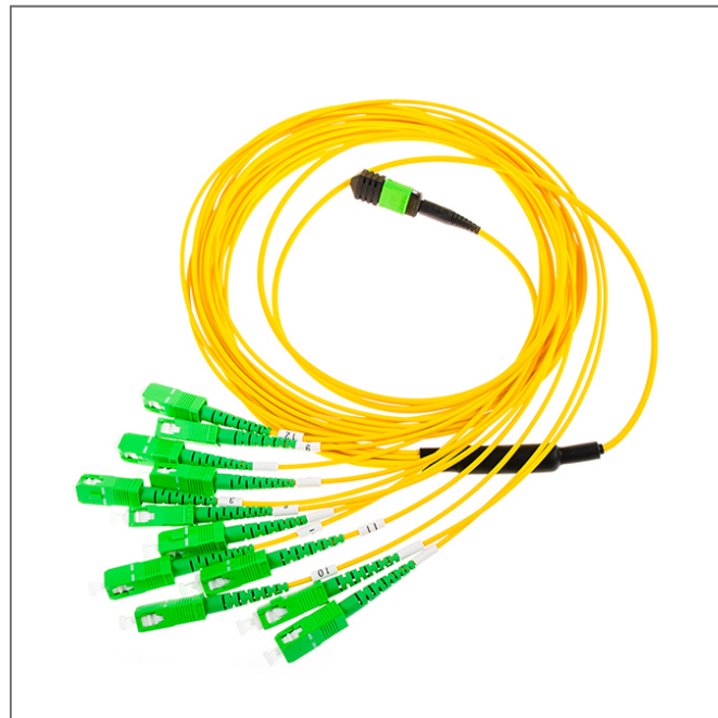
12cores MPO/MTP-12*SC/APC Simplex OS2
