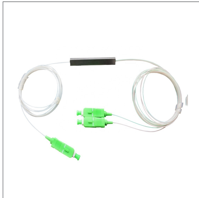
SC/APC 1x2 Steel Tube Mini type PLC 0.9mm
