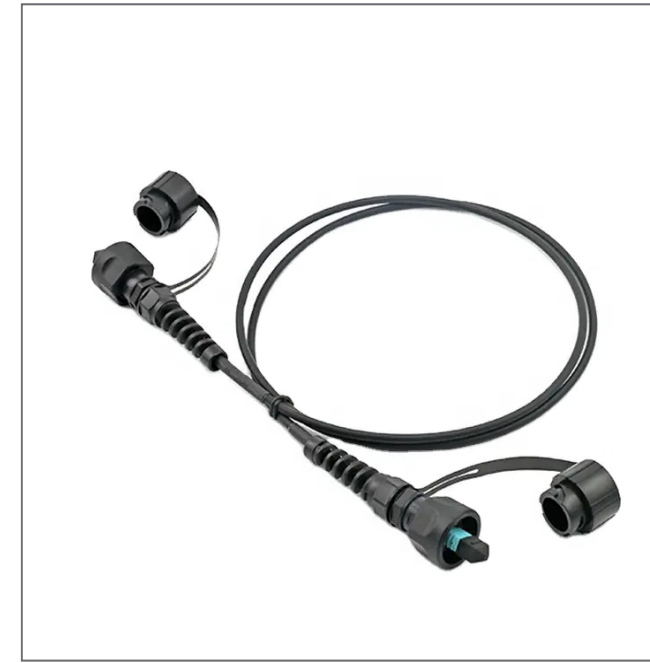
ODVA MPO/MTP-MPO/MTP 12cores
